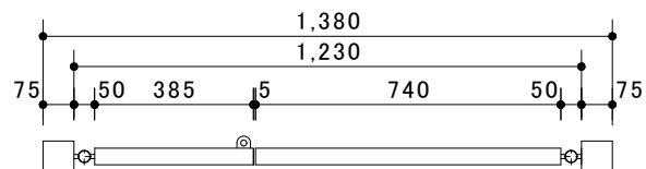
製品図
